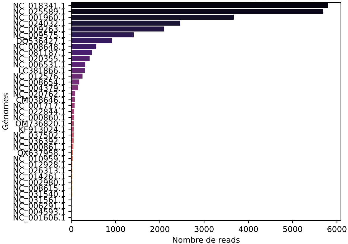
Reads par génome pour l'échantillon L2_4_CD2_S74_R1_001
