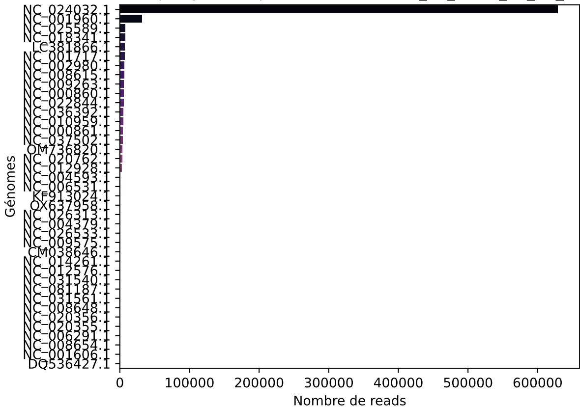
Reads par génome pour l'échantillon L3_13_MB11_S8_R1_001
