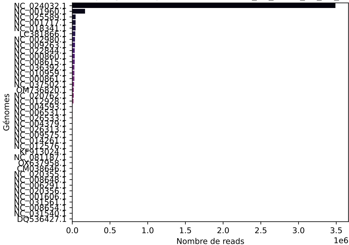
Reads par génome pour l'échantillon L3_14_MB10_S9_R1_001
