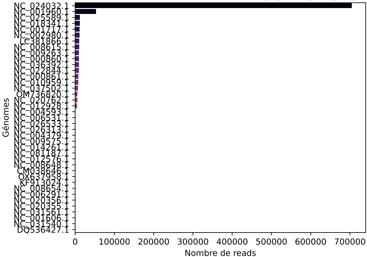
Reads par génome pour l'échantillon L4_1_MB14_S11_R1_001
