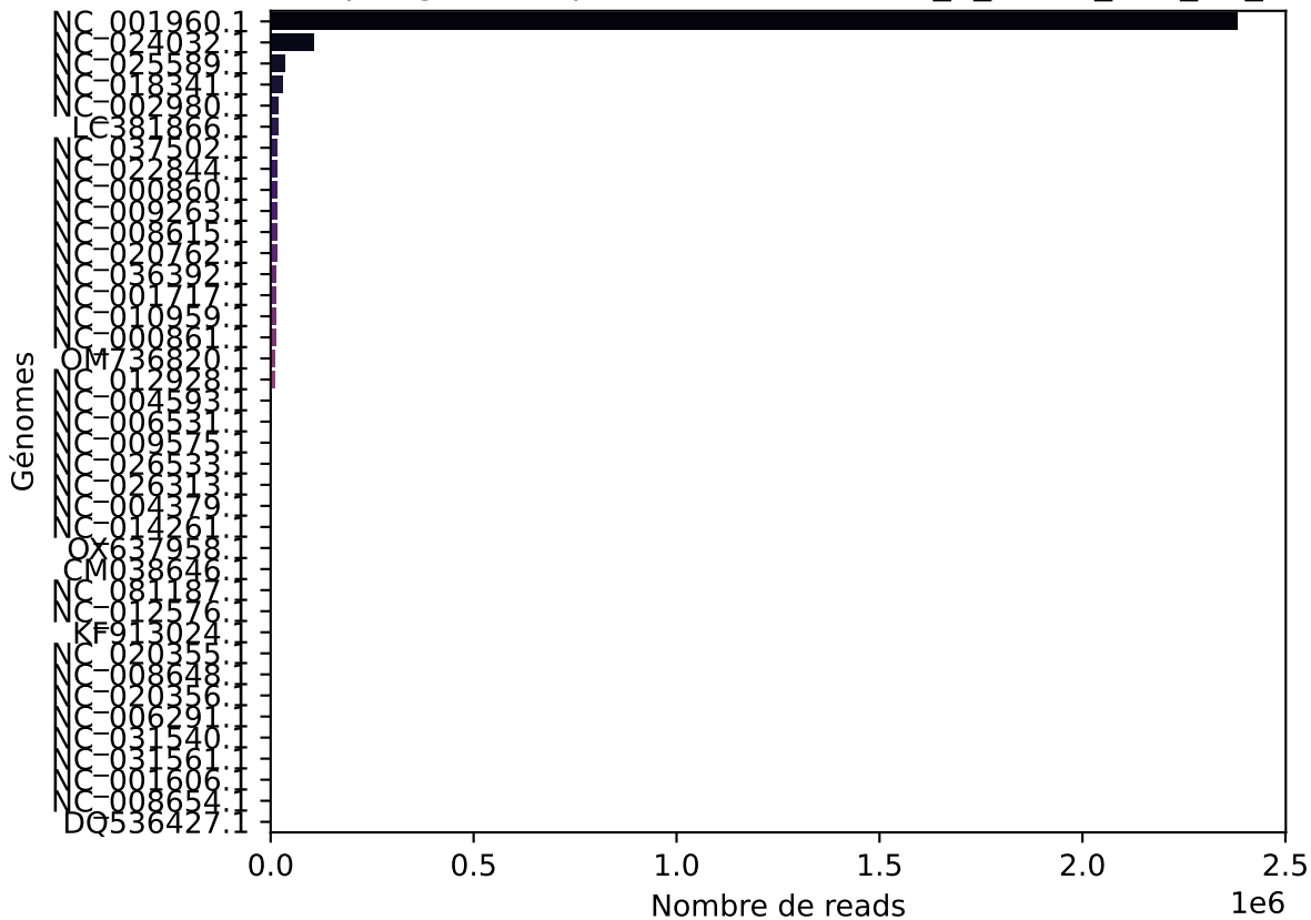
Reads par génome pour l'échantillon L5_5_MD10_S30_R1_001
